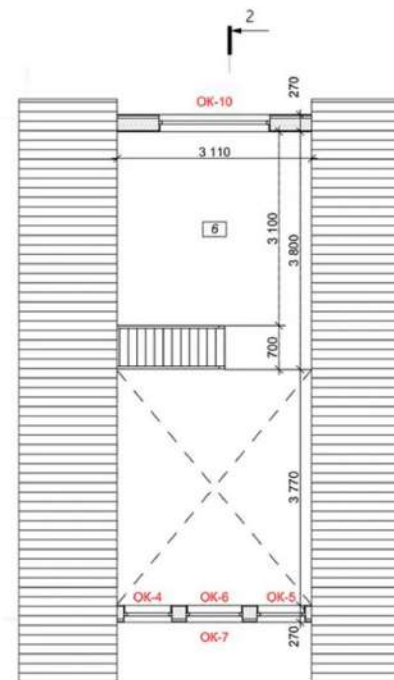
План антресоли
