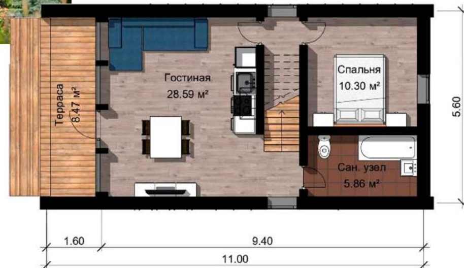
План 1 этажа
