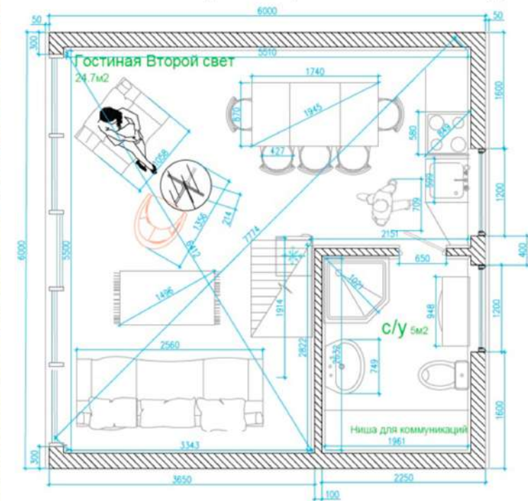
Планировка.Второй этаж. Две комнаты .
