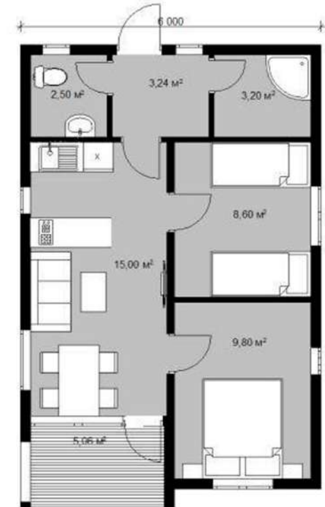
Варианты планировки
