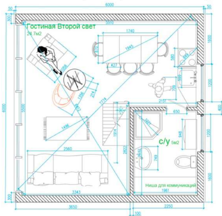
Планировка.Второй этаж. Две комнаты .
