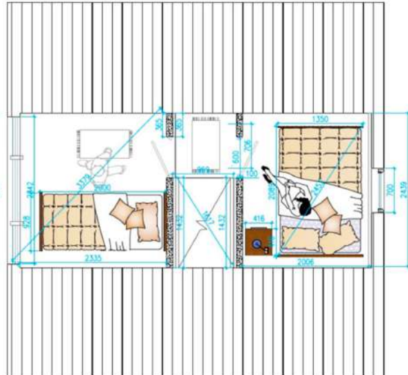
Планировка.Второй этаж. Две комнаты .
